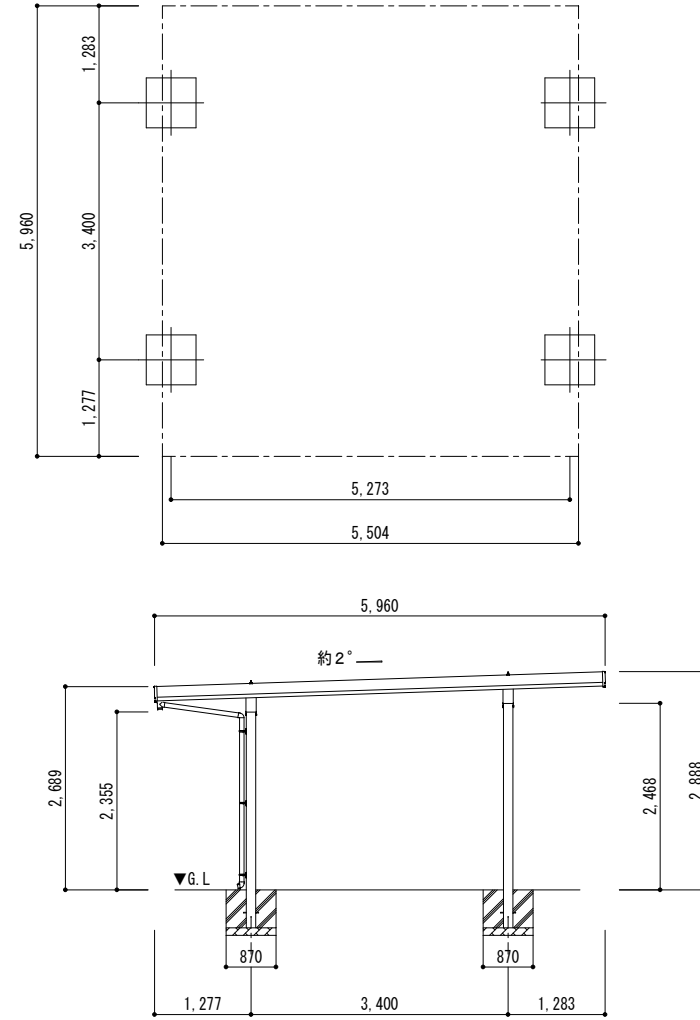
■基礎配置図
