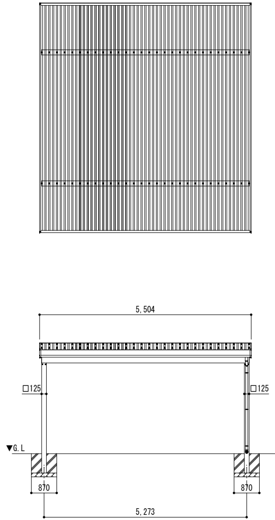
■姿図
